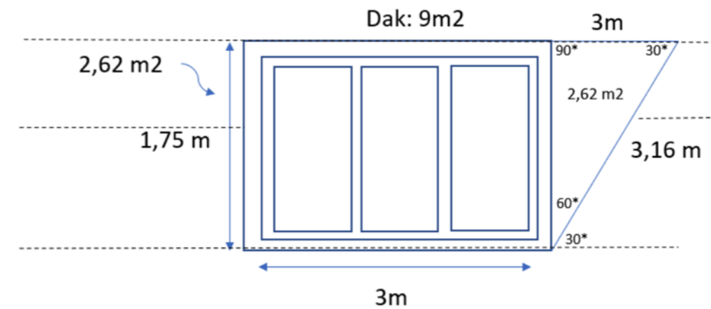
Afbeelding 2: Dimensies dakkapel.
